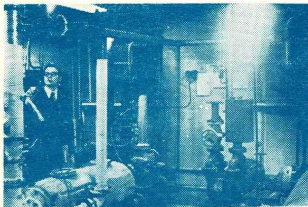
Установка по исследованию процесса сушки хлористого калия.
